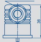
Pg 9 DIN 43 650
